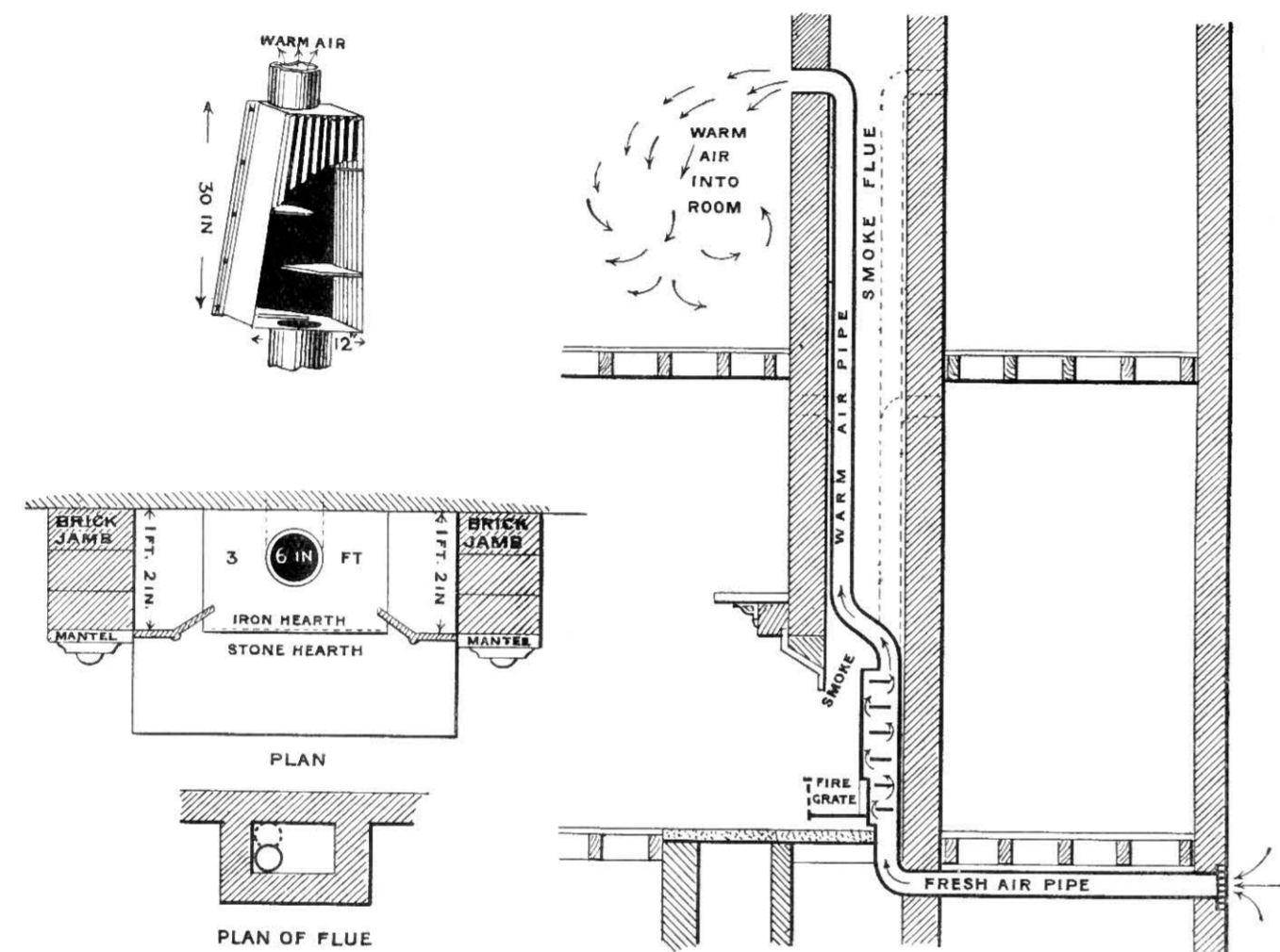
Fig. 476.—Shorland's Calorigen.
