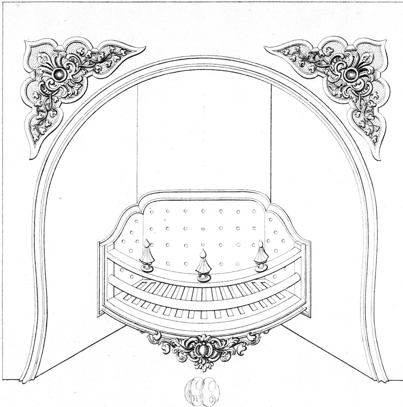
REGISTER STOVE N° 181.
